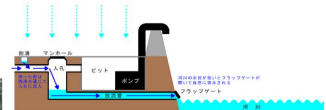
排水ポンプイメージ
