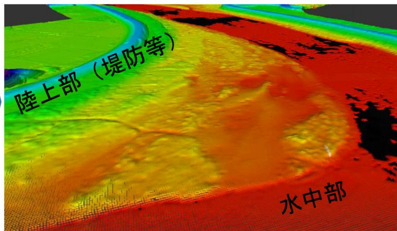
河川の三次元計測(イメージ)
