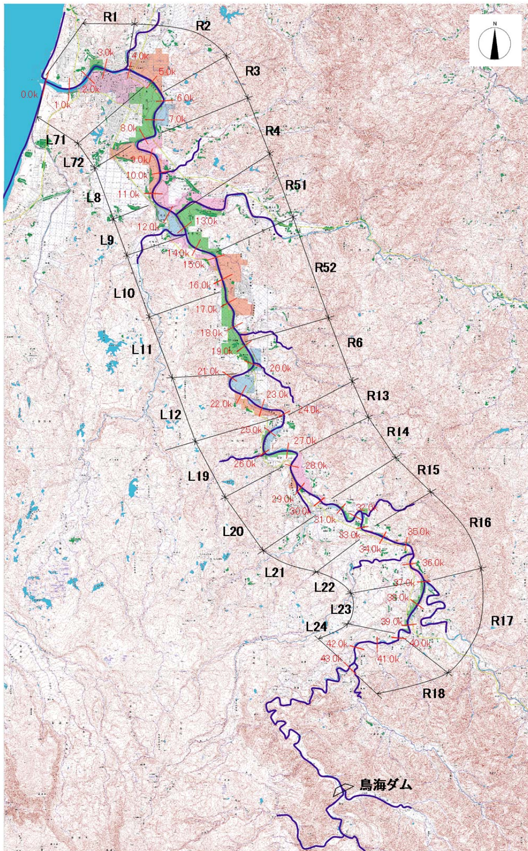
様式-1 氾濫ブロック分割図
