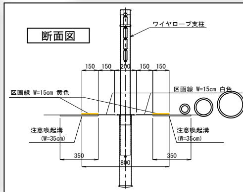
中央にワイヤーロープを設置し、より安全に
