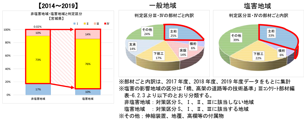
図 4 - 4 一般地域・塩害地域別の橋梁判定区分及び判定区分Ⅲ・Ⅳの部材ごと内訳
