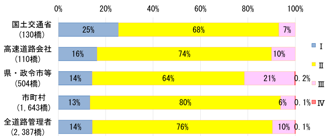
図3-2 2019年度の判定区分の割合(橋梁)
