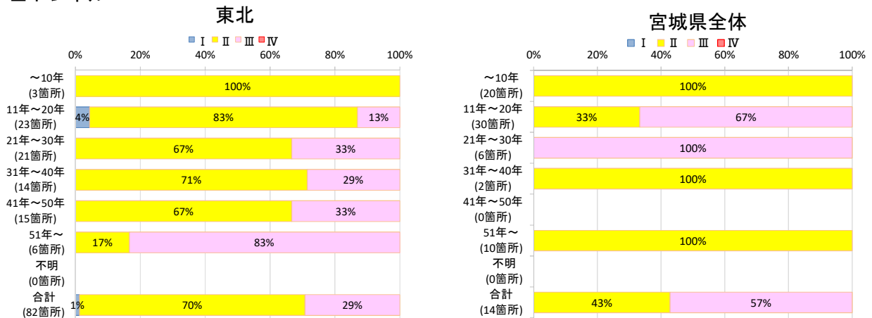
図6-17 建設年数別の判定区分の遷移状況
