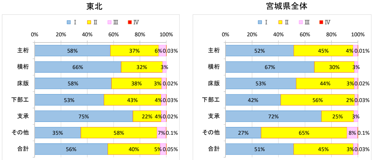
図6-2-1 部材ごとの判定区分【一般地域】
