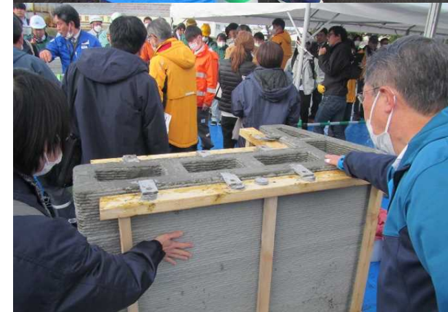
3Dプリンタで製作したコンクリート構造物を見たり触れたりする参加者
