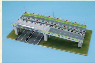
作品名 クリア歩道付PC中空床版橋 （耐震構造） 福島県立福島明成高等学校 環境土木科 鈴木 智弘（3年） 清野 隼（3年）
