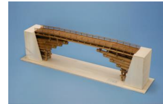
作品名 猿橋 宮城県古川工業高等学校 土木情報科 杉山 晴香（2年） 須藤 菜美（2年）
