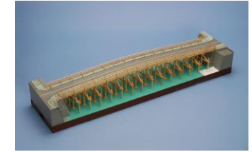
作品名 渡月橋 宮城県上沼高等学校 農業技術科 西條 伸也（3年）
