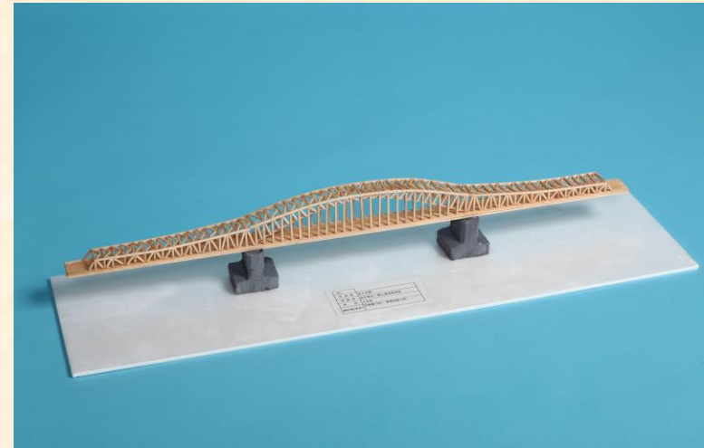
作品名 北上大橋 学校名 岩手県立一関工業高等学校 学 科 土木科 製作者 古澤 勇 (3年) 菅原 加奈 (3年)
