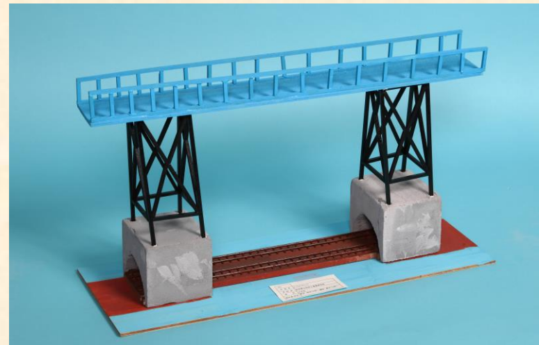
作品名 ミックスブリッジ 学校名 秋田県立秋田工業高等学校 学 科 土木科 製作者 鈴木 祐太 (3年) 鎌田 貢平 (3年)
