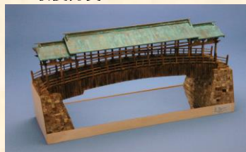
作品名 鞠橋 秋田県立大館工業高等学校 土木・建築科 日景 舞 (3年) 根田 溪介 (3年) 山脇 敬博 (3年)
