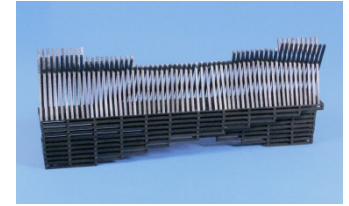
作品名 雪国橋 秋田県立秋田工業高等学校 土木科 田澤 紫織 (3年)
