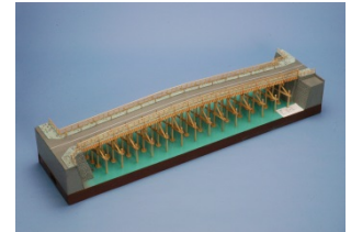
作品名 渡月橋 宮城県上沼高等学校 農業技術科 西條 伸也 (3年)
