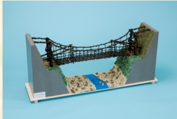
作品名 かずら橋 宮城県小牛田農林高等学校 我妻 恵一 菅原 敦 大槻 輝 佐藤 諒一
