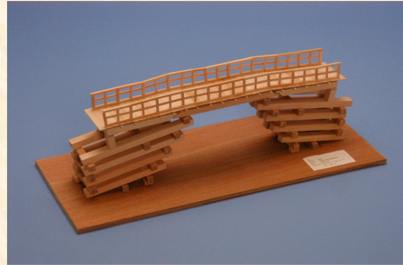
作品名 猿橋 学校名 福島県立磐城農業高等学校 学 科 緑地土木科 作成者 貝塚 拓 (3年) 伊藤 拓斗 (3年) 安井 将義 (3年)
