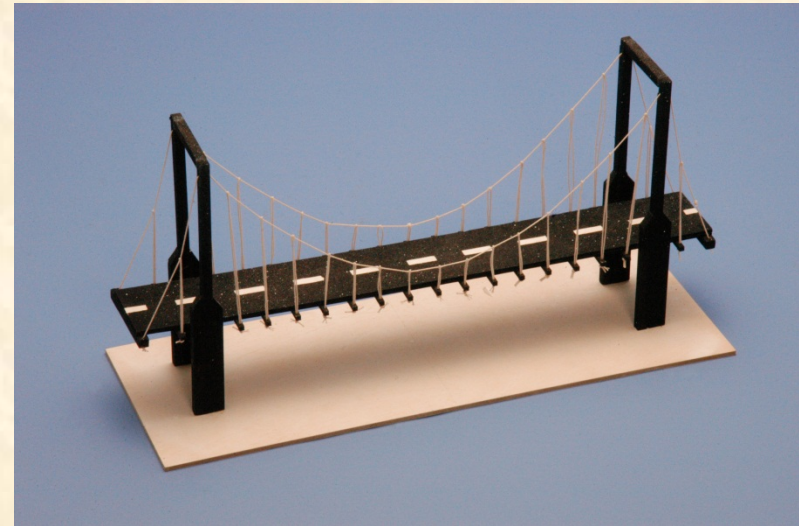
作品名 雪化粧した吊り橋 学校名 秋田県立秋田工業高等学校 学 科 土木科 作成者 門間 寿貴 (3年)
