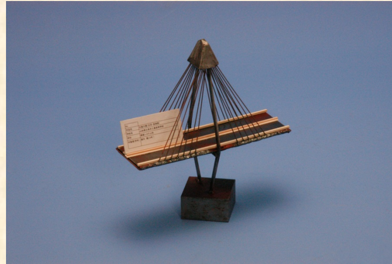
作品名 大島大橋 学校名 山形県立長井工業高等学校 学 科 環境システム科 作成者 高木 龍 (3年)
