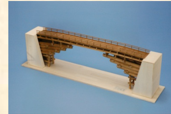
作品名 猿橋 宮城県古川工業高等学校 土木情報科 杉山 晴香 (2年) 須藤 菜美 (2年)
