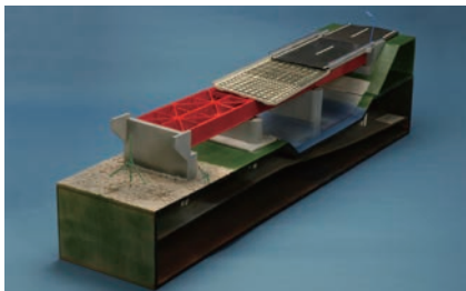
アイデア賞 | 3径間連続複合橋 構造模型 青森県立柏木農業高等学校 環境緑地科・土木コース 工藤 拓也 (2年) 後藤 瑤 (2年) 齋藤 啓大 (2年) 館山 晃佑 (2年) 福士 昂生 (2年) 村元 颯哉 (2年) 盛 悠輝 (2年)
