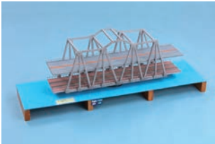
アイデア大賞 2位 フォート・マディソン有料橋 青森県立青森工業高等学校 都市環境科 阿保 友唯 (3年) 小枝日菜梨 (3年) 高橋 康太 (3年) 佐々木将人 (3年) 豊嶋 椎麻 (3年)
