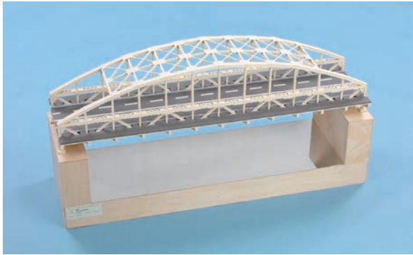
最優秀賞 ストラクチャル大賞 ビジュアル大賞 アイデア大賞 3位 開運橋(二度泣き橋) 秋田県立横手清陵学院高等学校 総合技術科 川越 天磨 (2年) 菊池 悠貴 (2年) 高橋 沙羅 (2年) 高橋 柚月 (2年)
