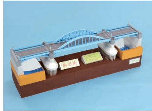
最優秀賞/プレゼンテーション賞 駒形橋 秋田県立秋田工業高等学校 土木科 鎌田 朔羅 (3年) 熊谷 拓人 (3年) 小玉 碧海 (3年) 杉本 真弥 (3年) 武内 大和 (3年) 細川 優 (3年)
