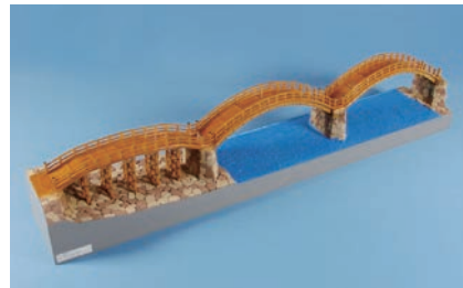
優秀賞 | 錦帯橋 宮城県小牛田農林高等学校 農業技術科 農業土木コース 古内 聡 (2年) 大和田 俊太 (2年) キガンテ ニコ (2年)
