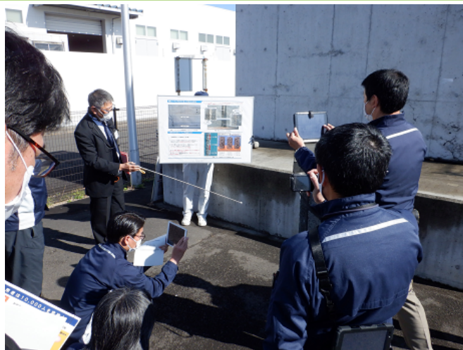
締固めの違いによる影響について
