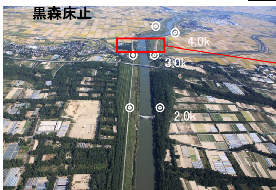
床止の改築
