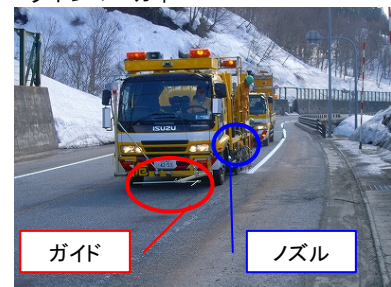
施工状況 (ラインマーカー車)
