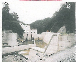
赤沢第3堰堤
