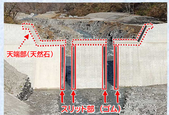
主堰堤 (ウラ)
