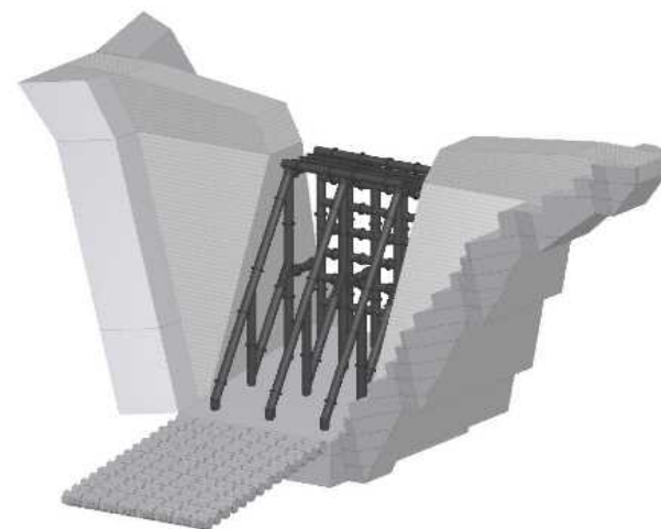
水沢第3砂防堰堤
