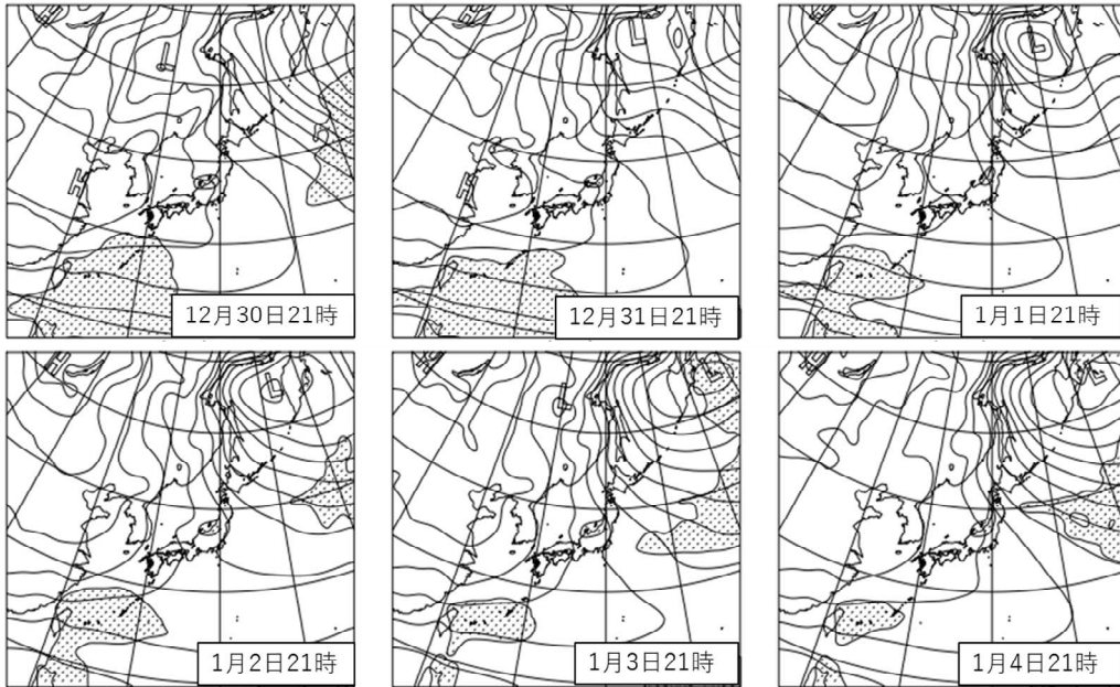
地上予想天気図 (令和4年12月30日～令和5年1月4日) ※ハッチは降水域
