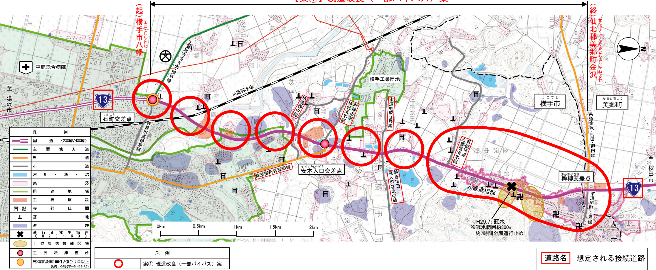
【案①】現道改良(一部バイパス)案
