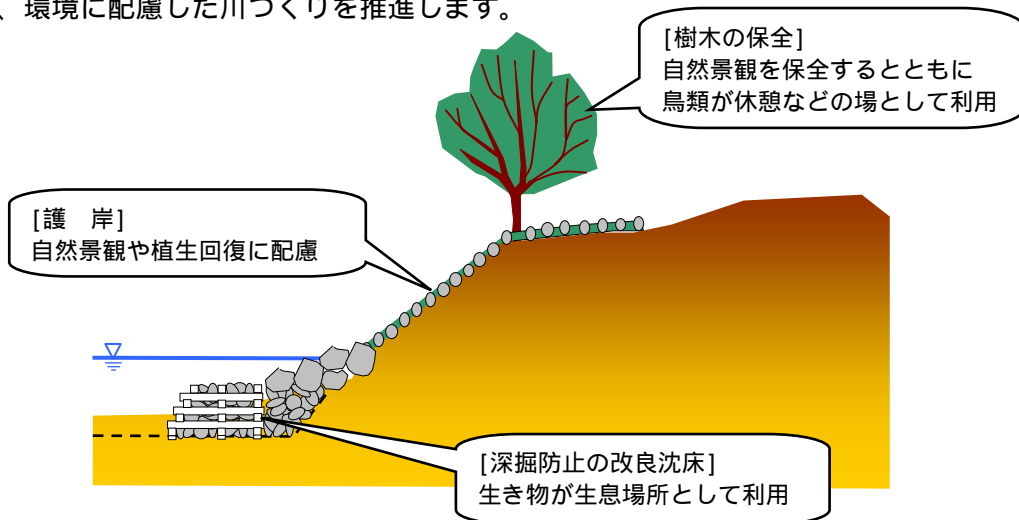
図 5.12 護岸の設置における多自然川づくりのイメージ
