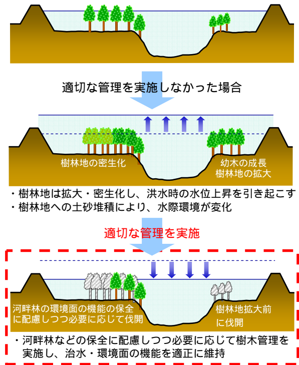
図 5.16 樹木管理のイメージ（断面図）
