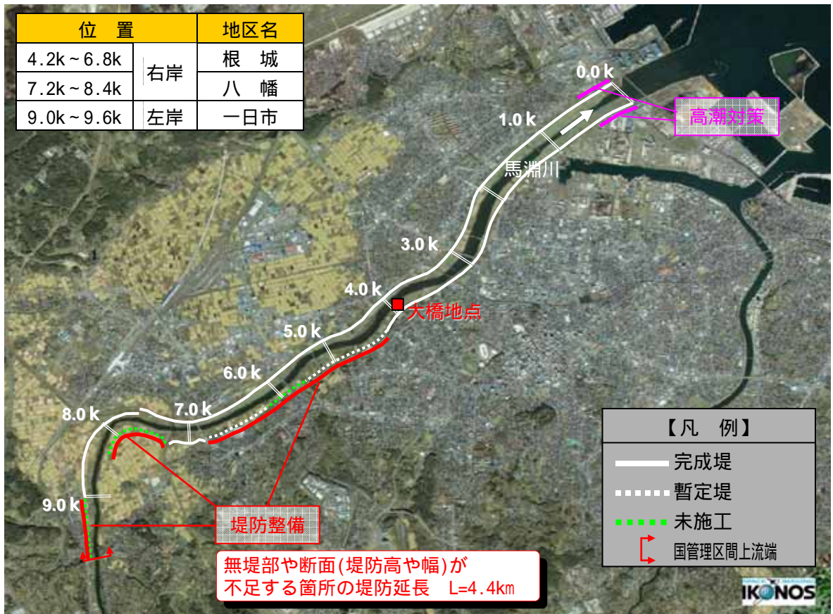
図 5.3 堤防の量的整備位置(平成 21 年 3 月時点)
