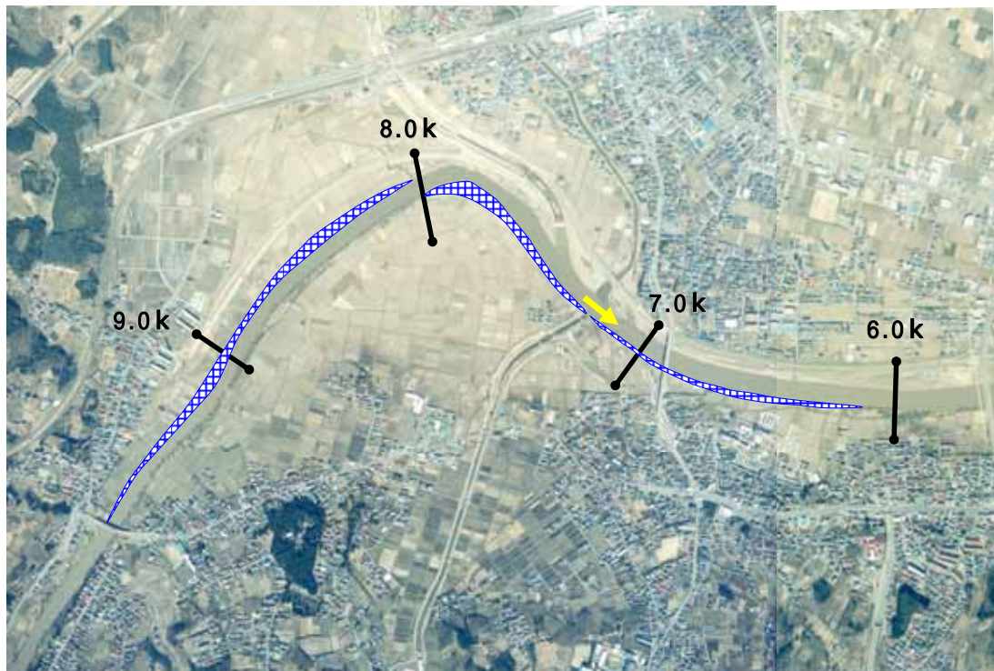
図 5.8 河道掘削位置（平成 21 年 3 月時点）
