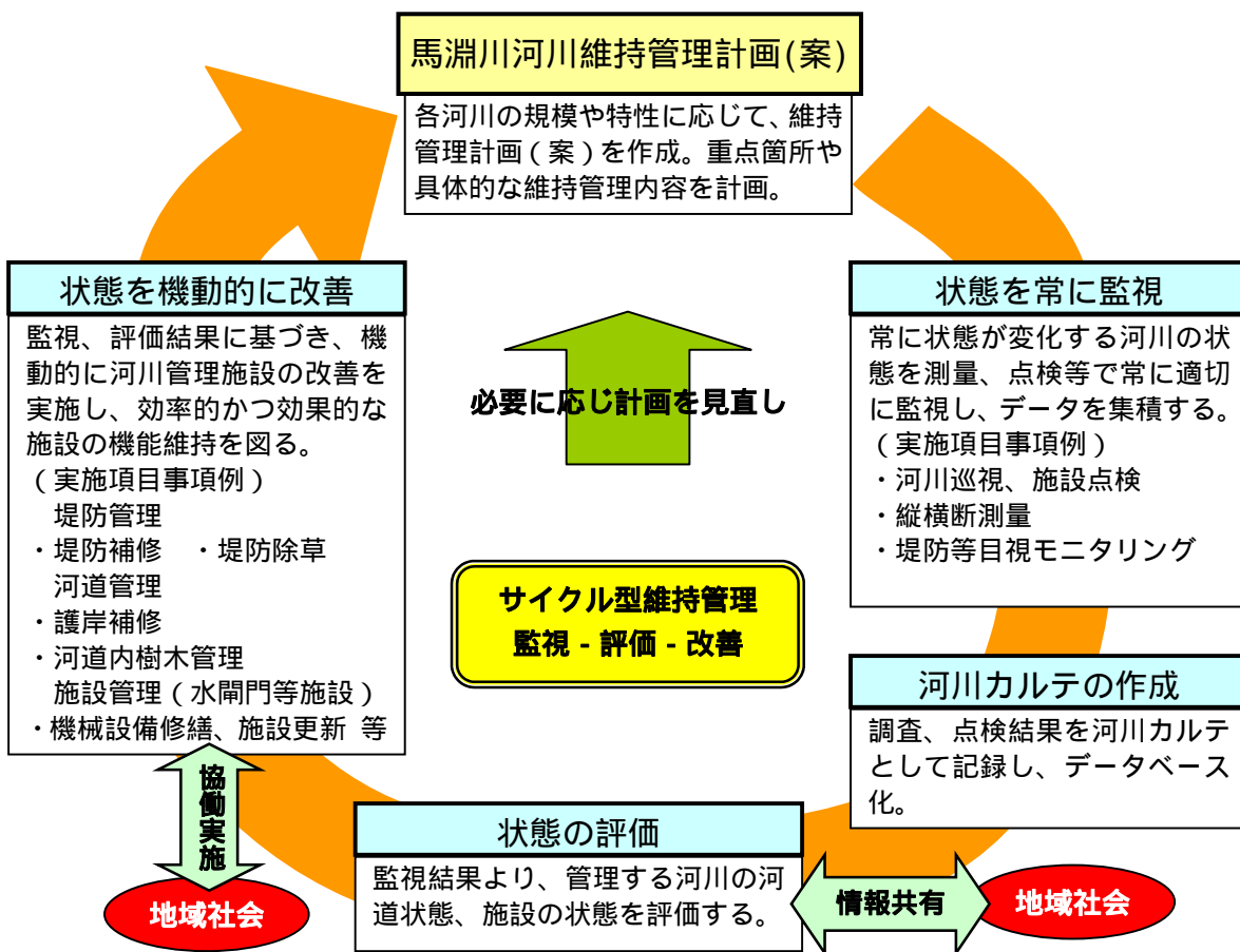
図 5.14 サイクル型維持管理のイメージ
