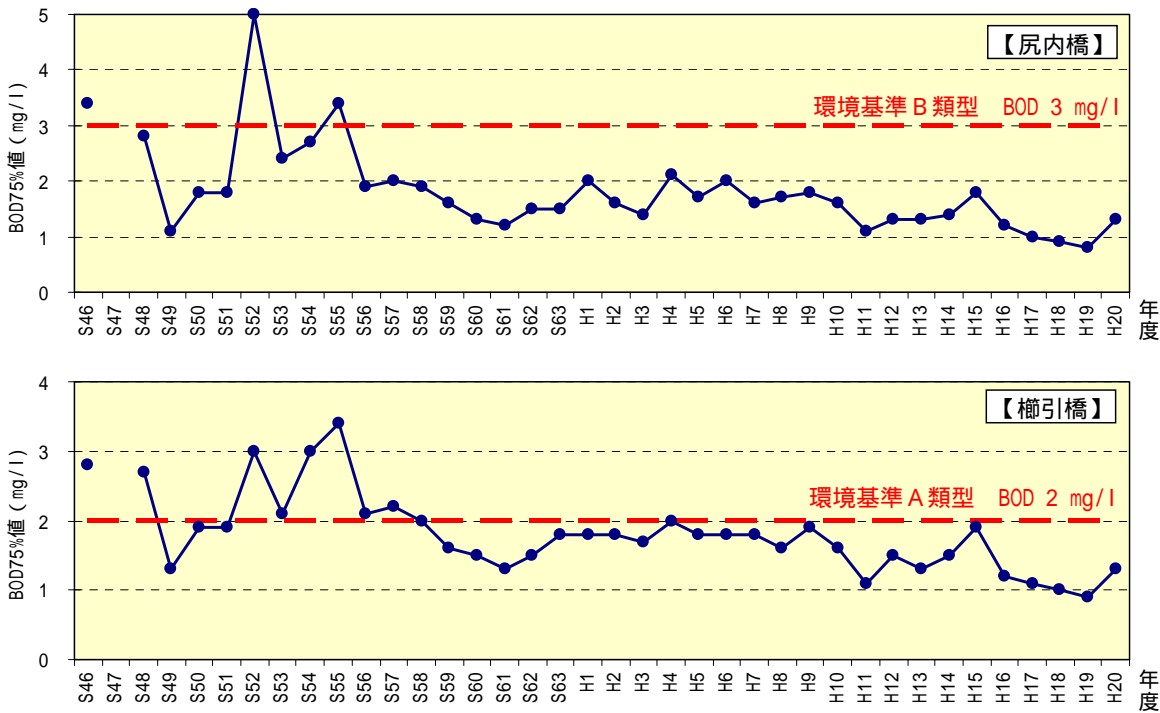
図 3.16 各環境基準点における水質経年変化(BOD75%値 2 )
