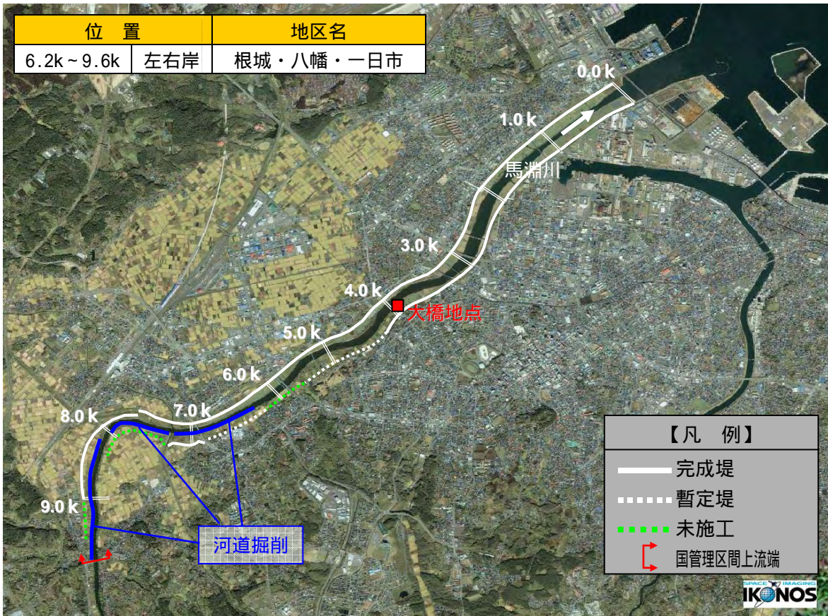
図 5.8 河道掘削位置（平成 21 年 3 月時点）
