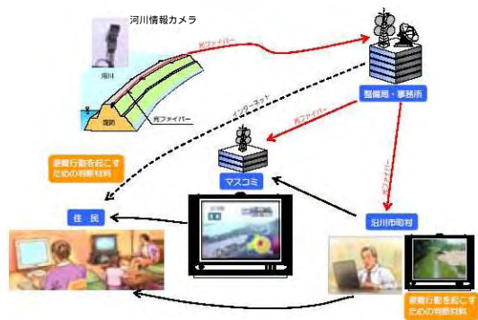
図 5.18 洪水情報共有システム構成図
