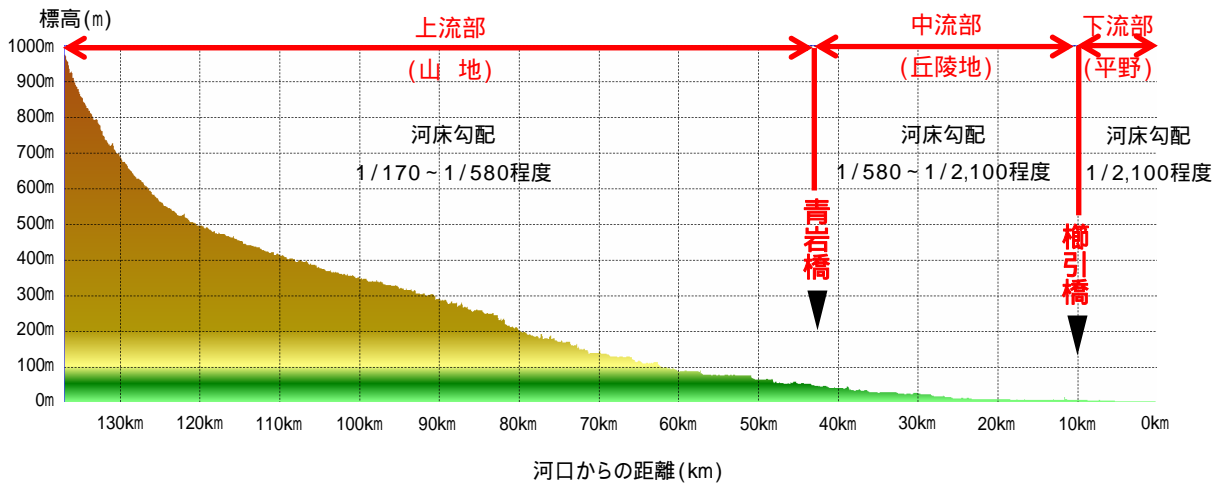
図 3.2 馬淵川河床勾配縦断図
