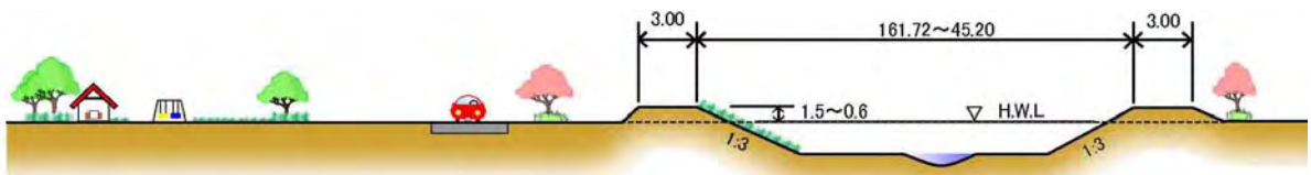
整備イメージ（馬淵川合流点～渡の葉橋の放水路）
