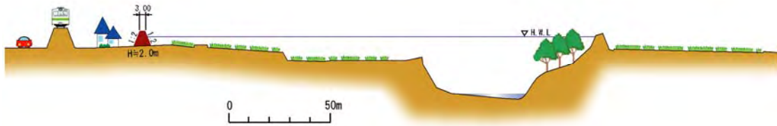
整備イメージ (横断面)
