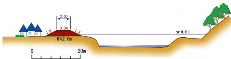
整備イメージ (横断面)
