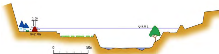
整備イメージ (横断面)
