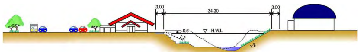
整備イメージ（渡の葉橋～滝谷橋付近）
