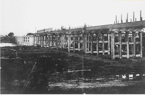
昭和4年10月 乾橋架替工事 (51cm x 42cm)
