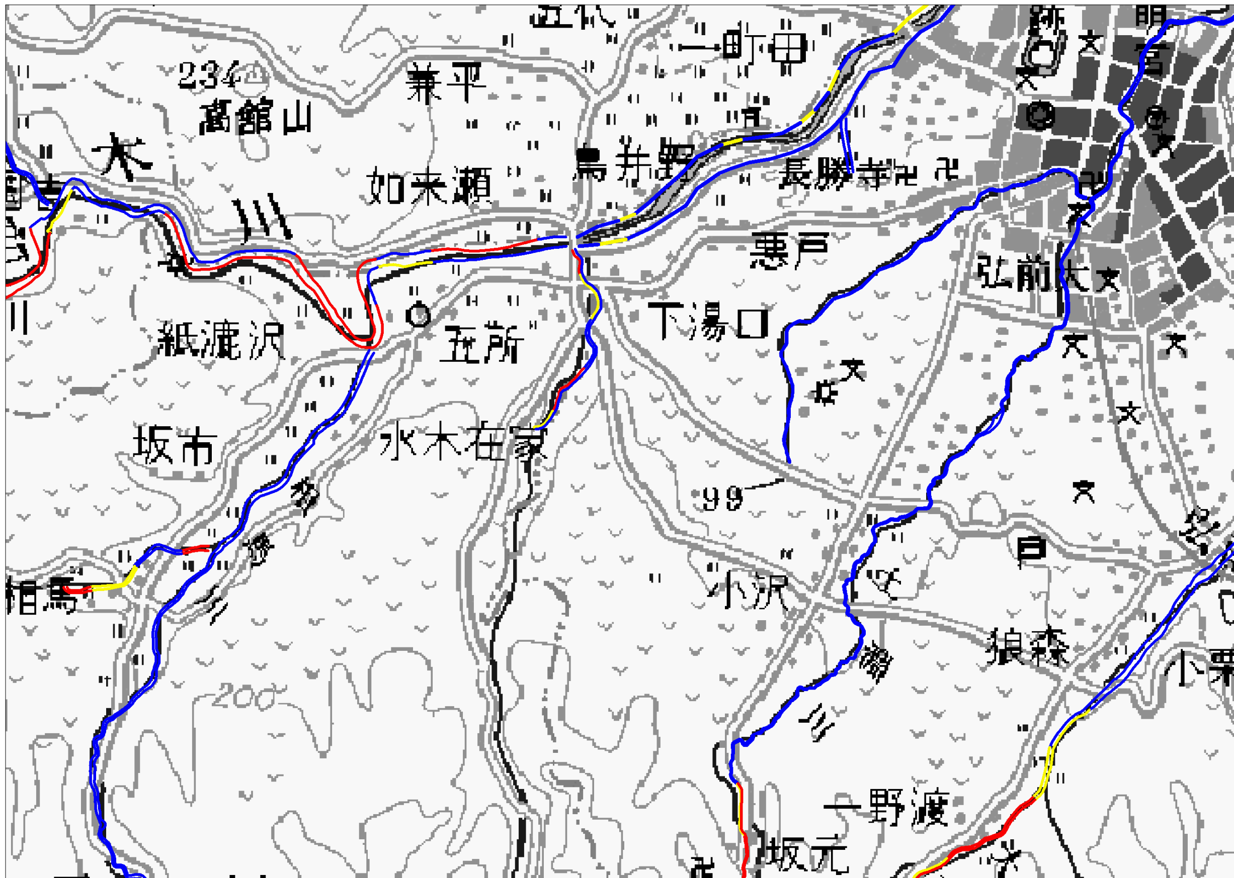
岩木川水系治水安全度評価図（拡大図 15）
