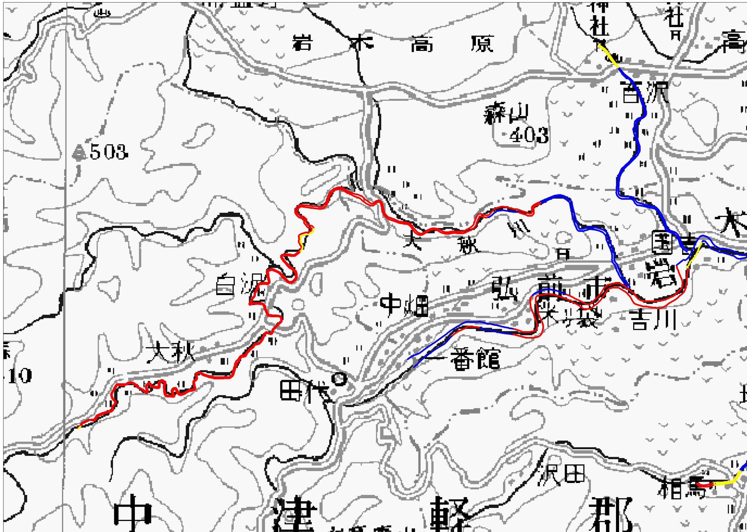
岩木川水系治水安全度評価図（拡大図 17）
