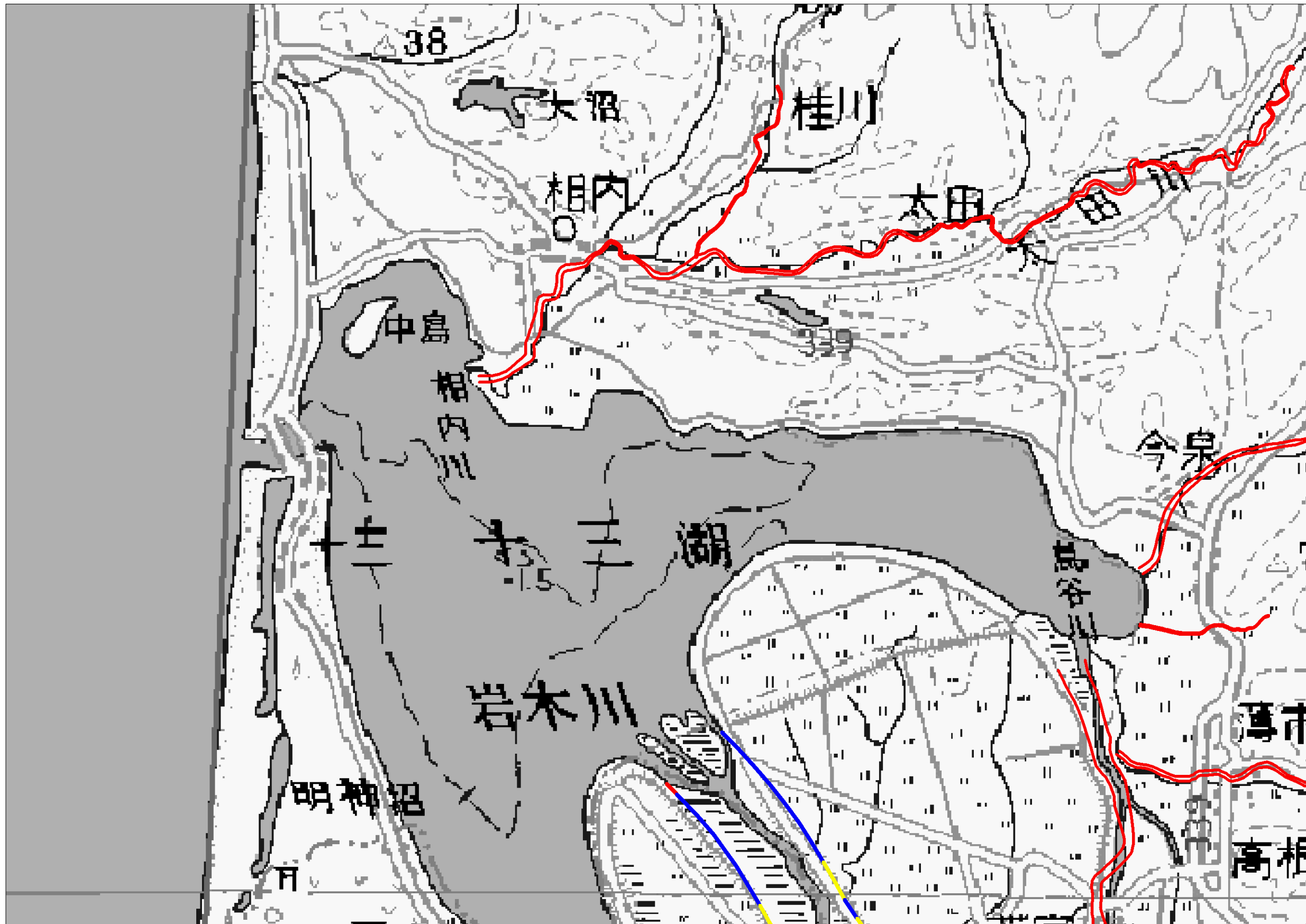
岩木川水系治水安全度評価図（拡大図 1）
