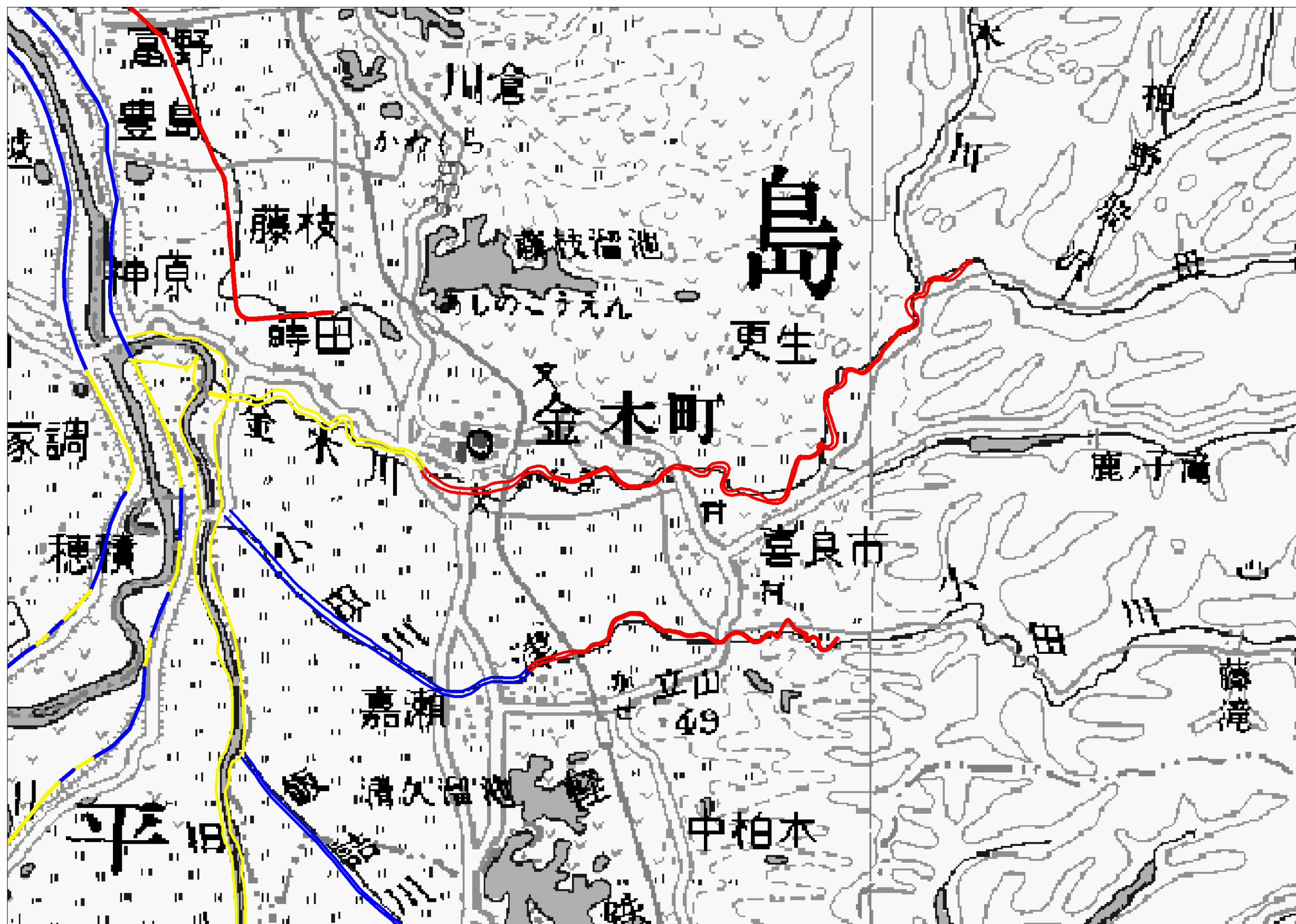
岩木川水系治水安全度評価図（拡大図 5）
