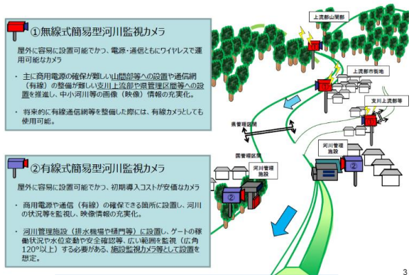
簡易型河川監視カメライメージ
