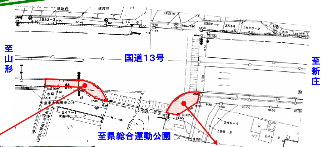
補修前の歩道状況です。 すり付け勾配は約20%（11度）ときつく、 シニアカーの通行や積雪時の歩行などに 支障がありました。
