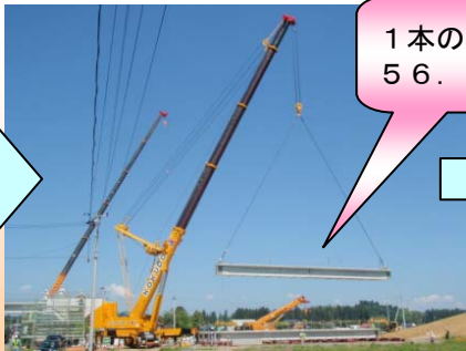
橋桁を1本ずつ架設します
