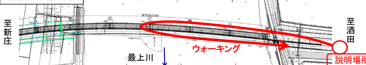
(仮称)古口大橋 平面図
