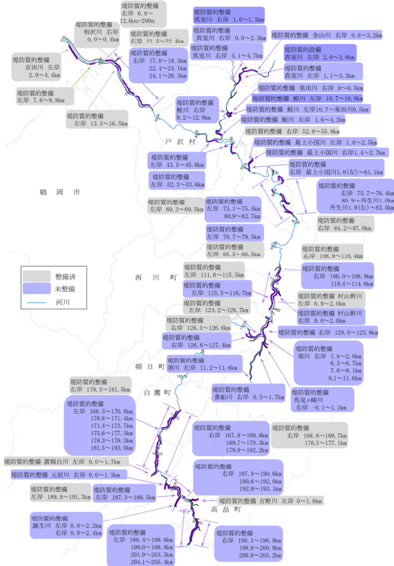
図 5-20 堤防質の整備位置図
