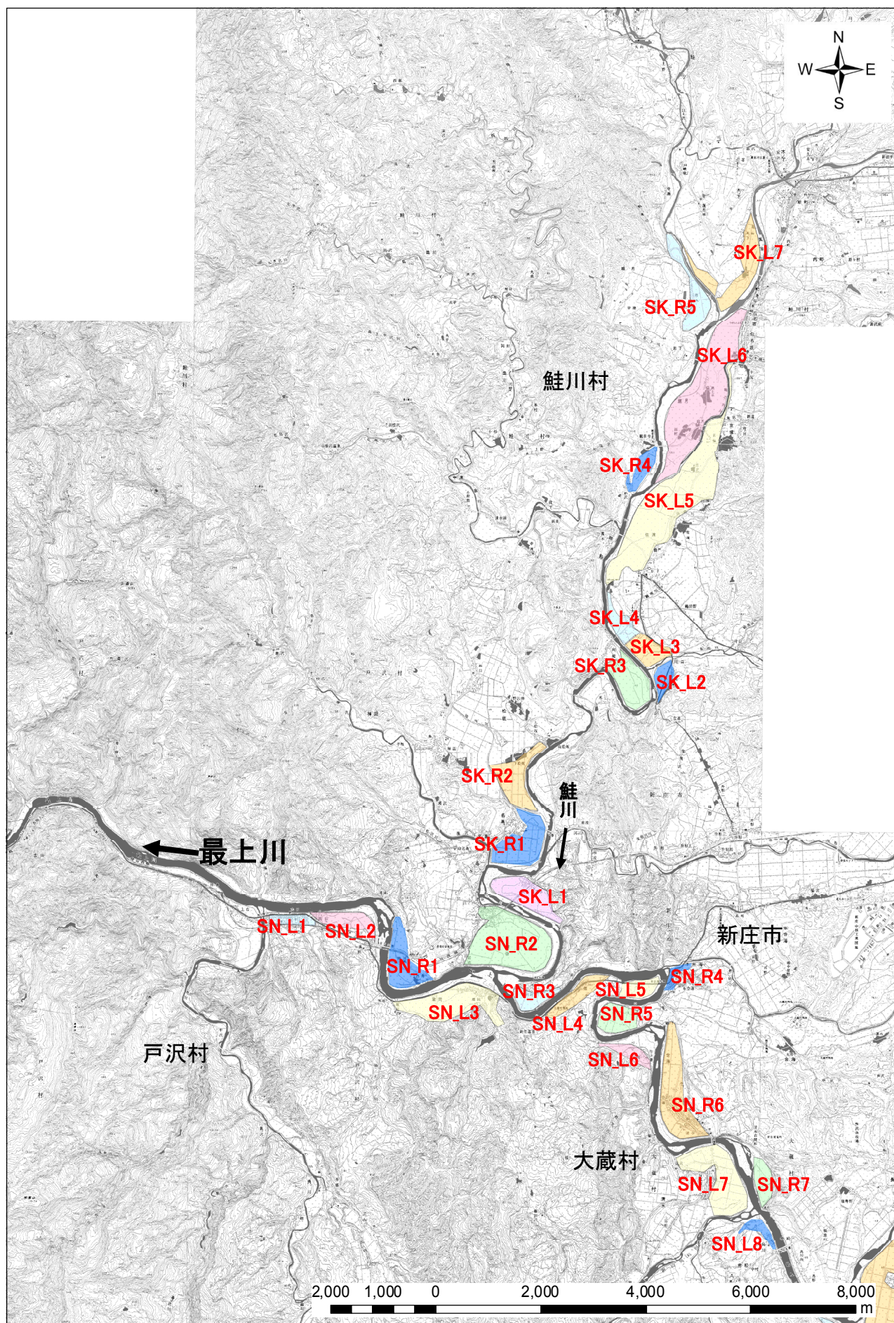
様式-1 氾濫ブロック図 最上川 (4/9)
