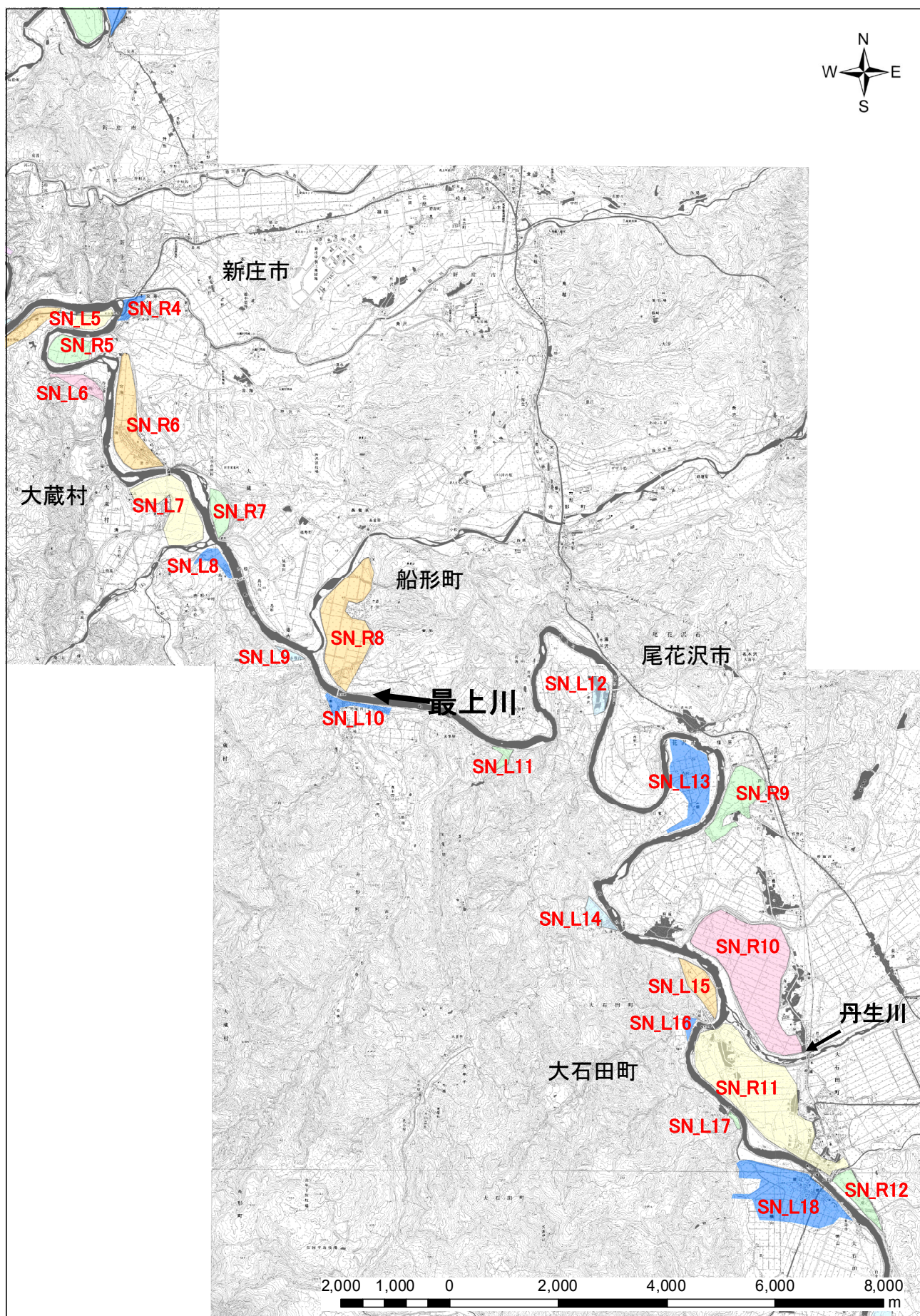
様式-1 氾濫ブロック図 最上川 (5/9)
