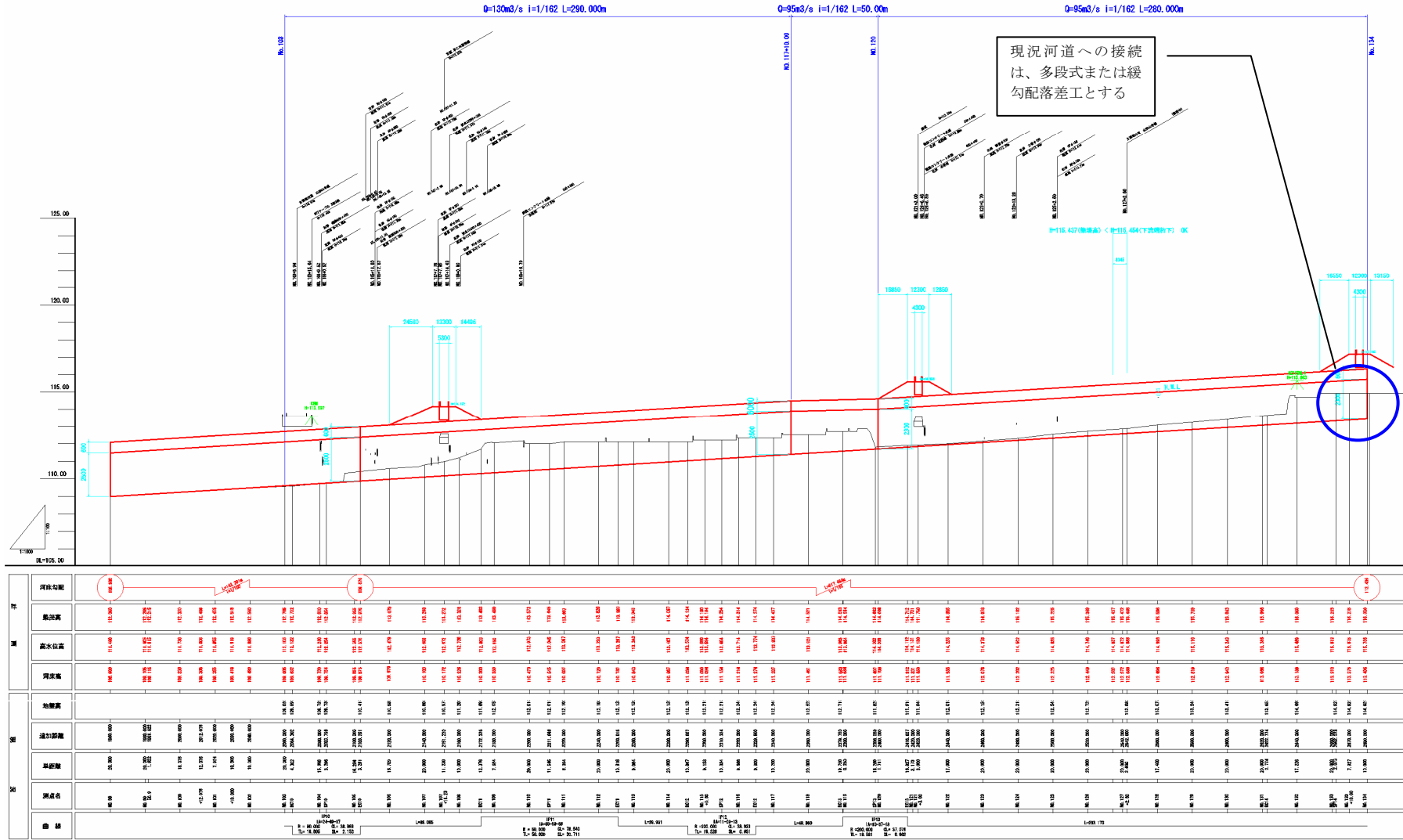
図-1.2 野呂川「延伸区間」計画縦断面図
