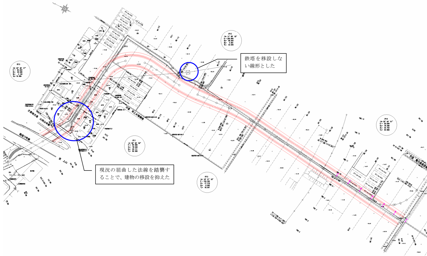
図-1.1 野呂川「延伸区間」計画平面図
