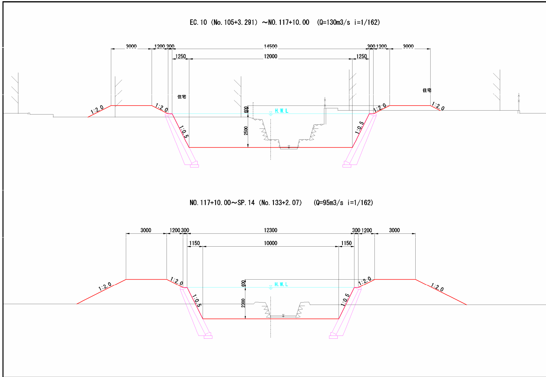
図-1.3 野呂川「延伸区間」標準断面図
