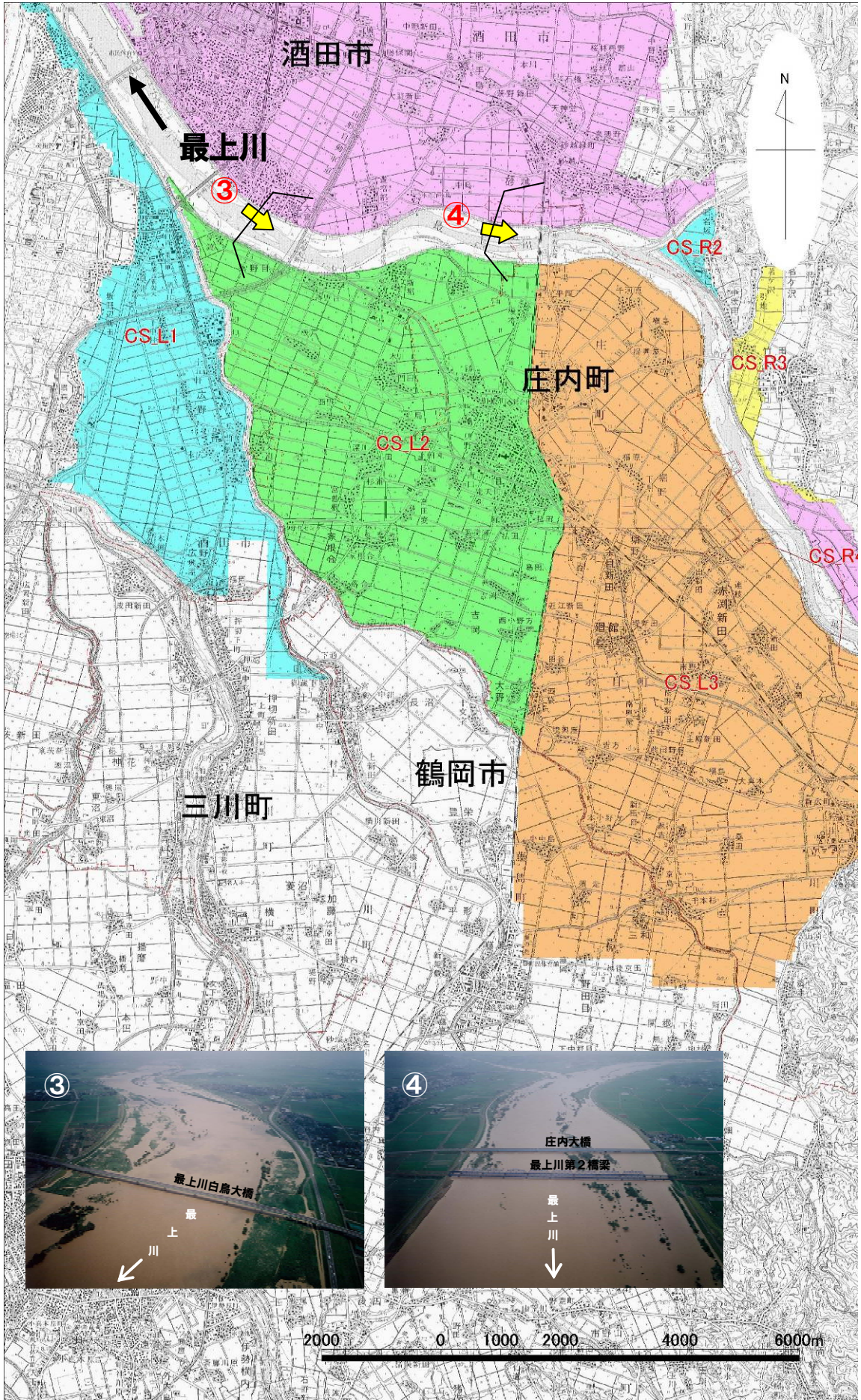
様式-1 氾濫分割図 最上川(2/9)
