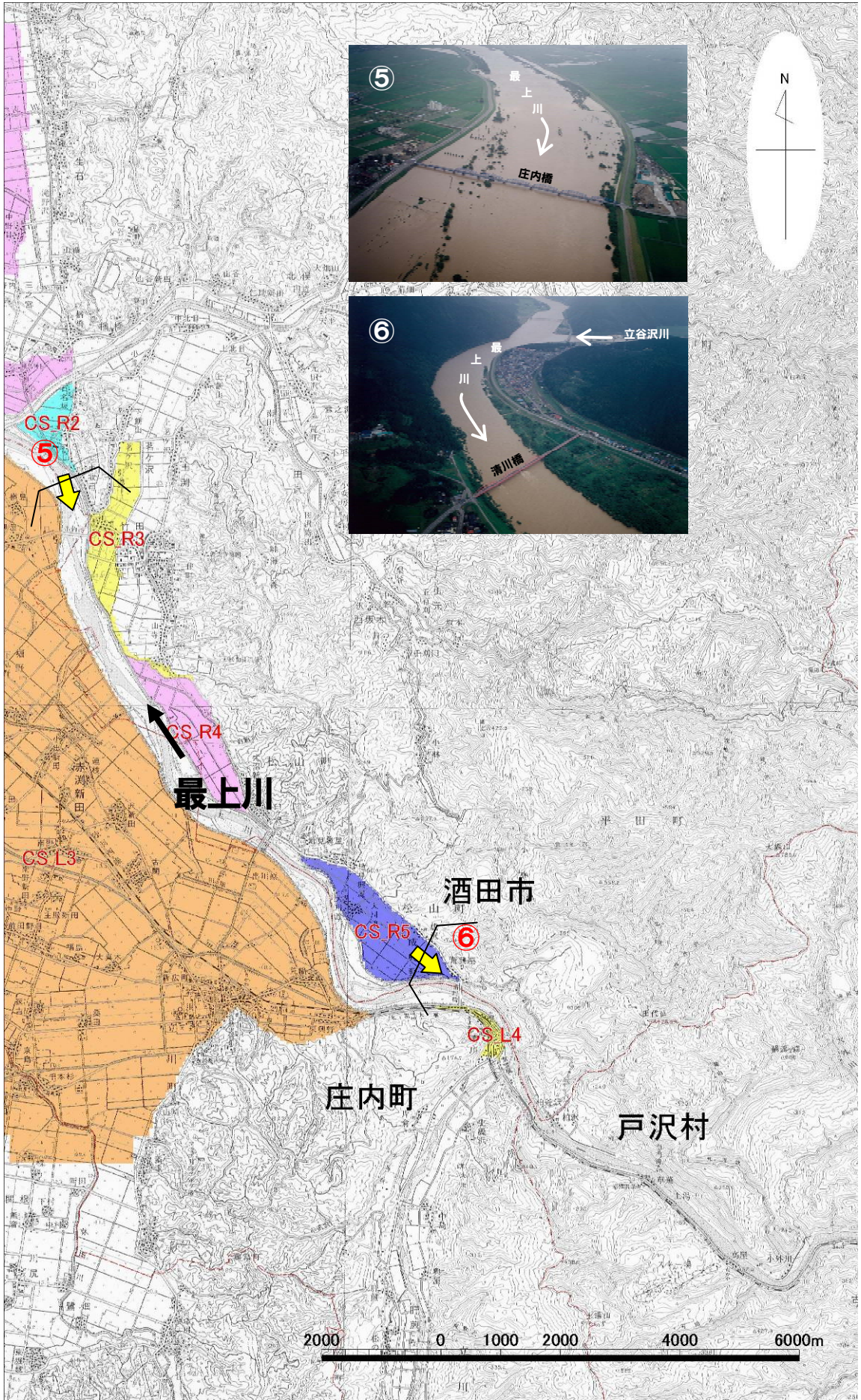
様式-1 氾濫分割図 最上川(3/9)
