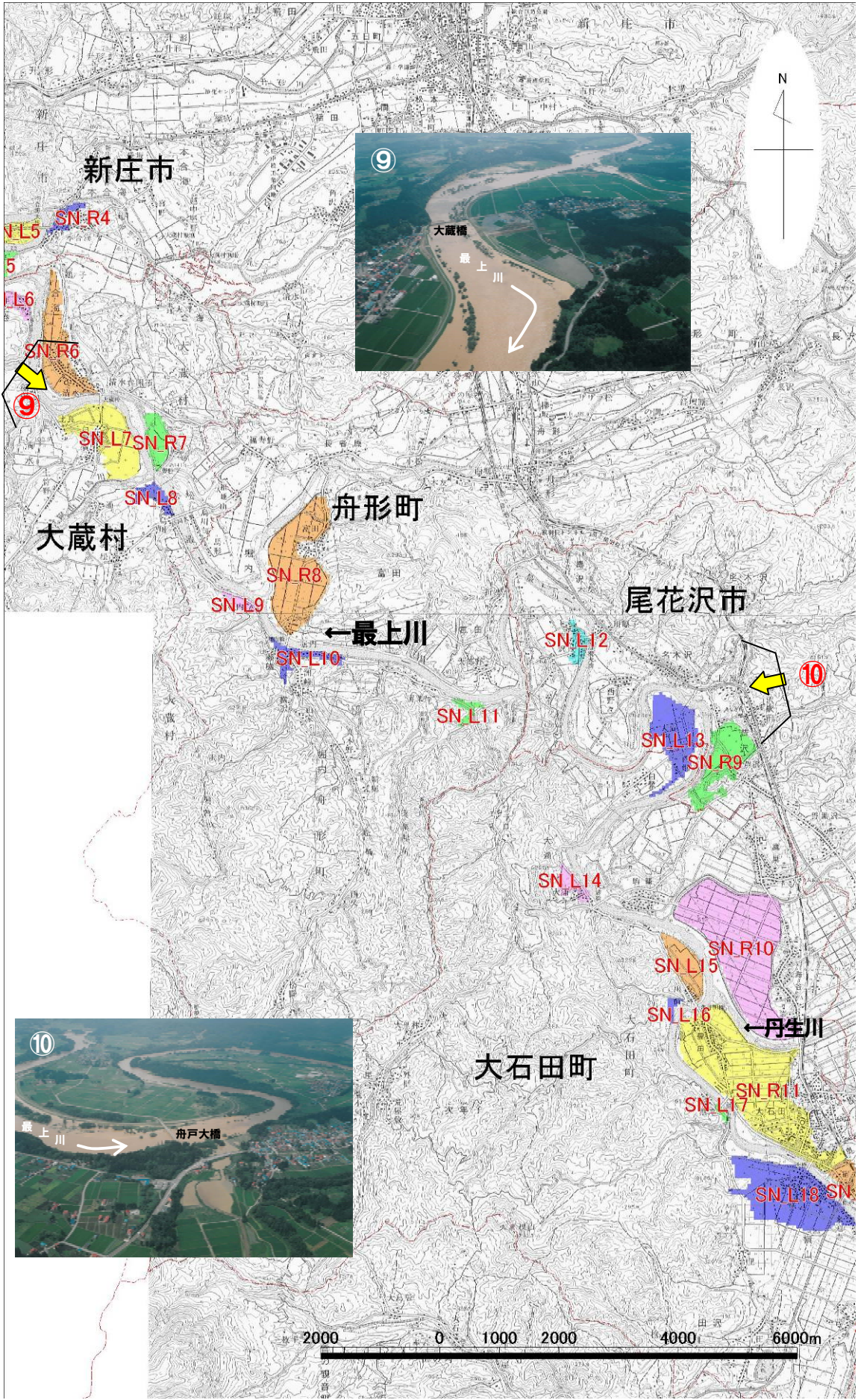
様式-1 氾濫分割図 最上川(5/9)
