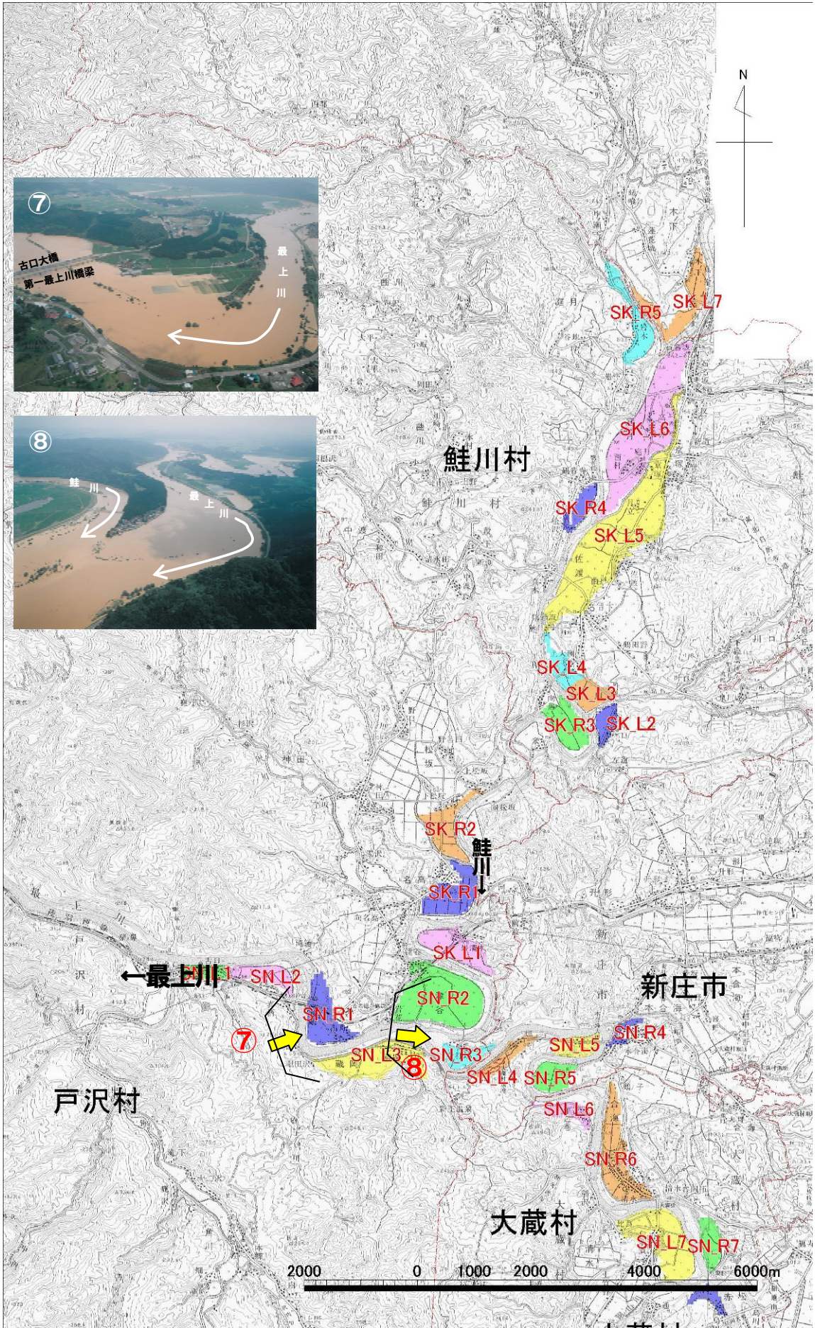
様式-1 氾濫分割図 最上川(4/9)
