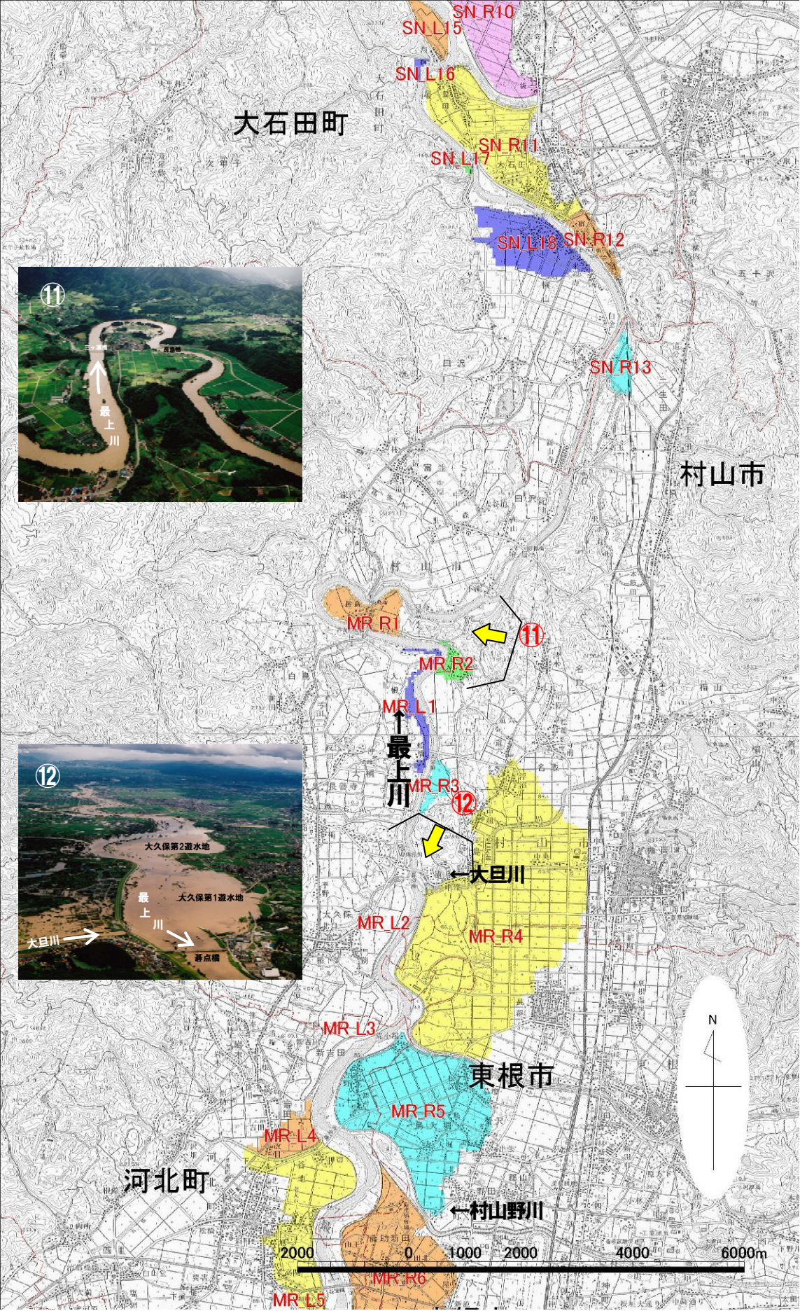
様式-1 氾濫分割図 最上川(6/9)
