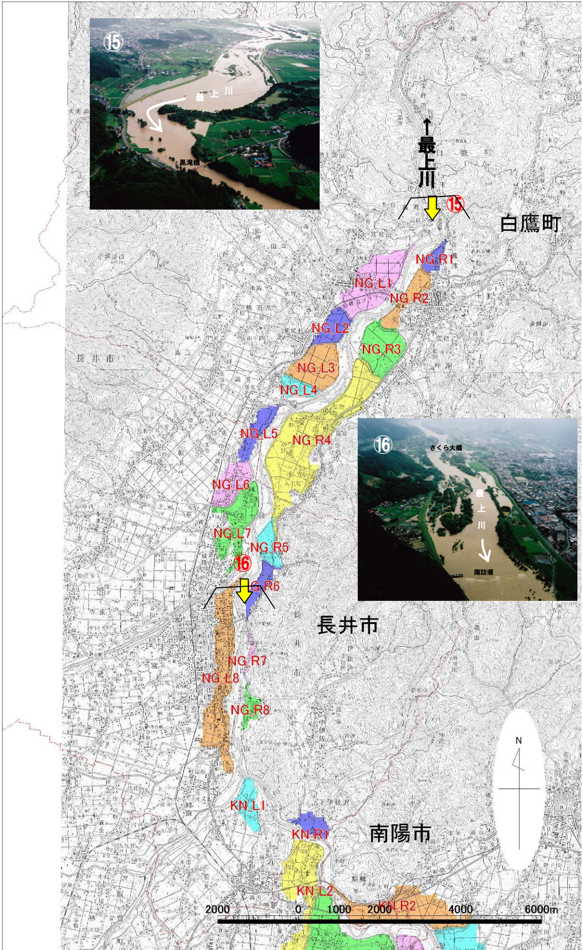
様式-1 氾濫分割図 最上川(8/9)
