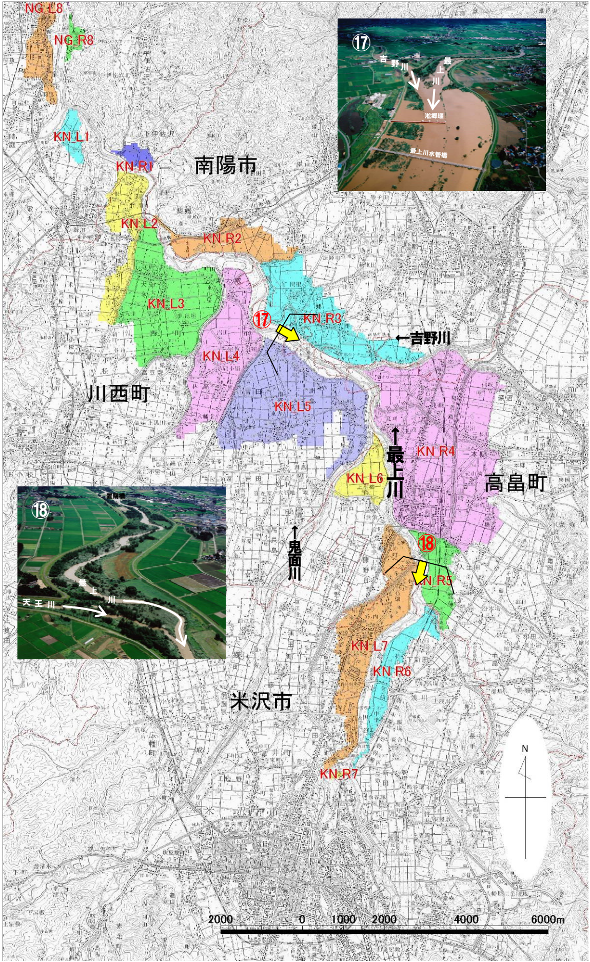
様式-1 氾濫分割図 最上川(9/9)
