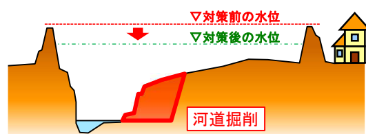
河道掘削(イメージ)
