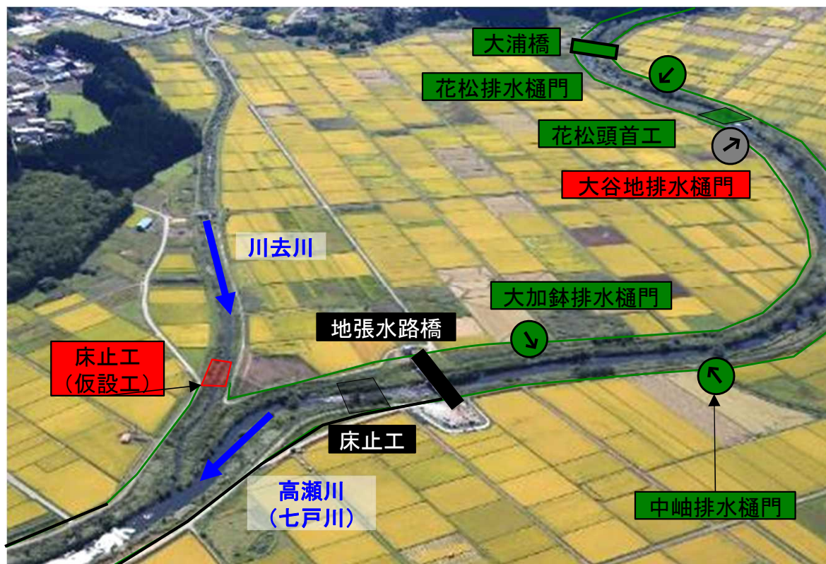
七戸川（高瀬川）改修事業
