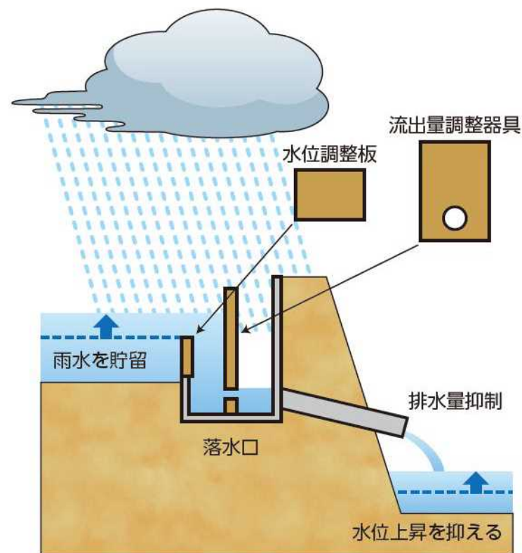
田んぼダム（イメージ）
