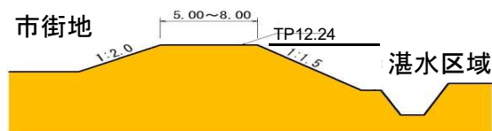
二線堤 横断面図
