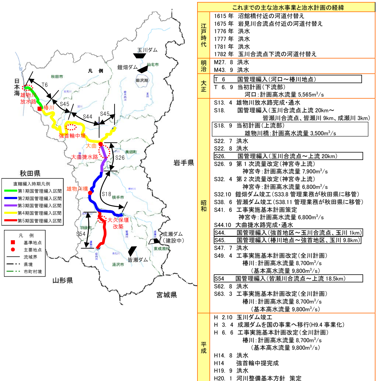
図 2.2-1 雄物川水系における改修計画の経緯及び事業区間位置図
