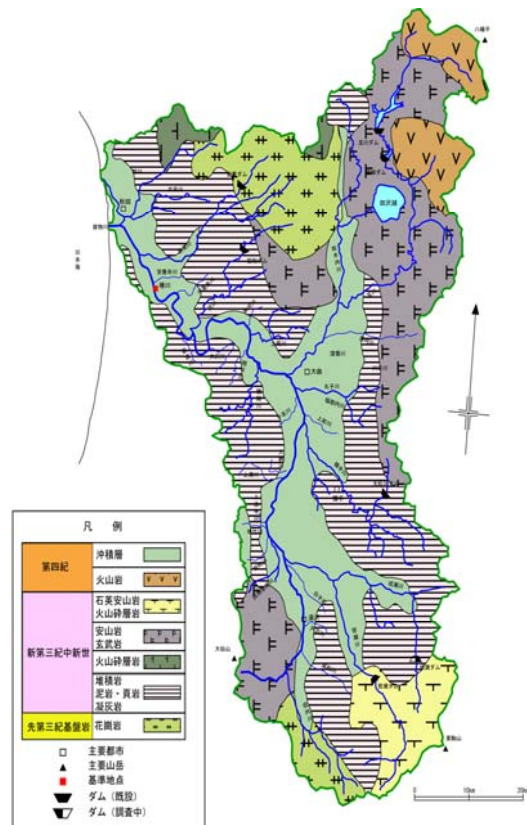
図 2.1-3 雄物川流域地質図
