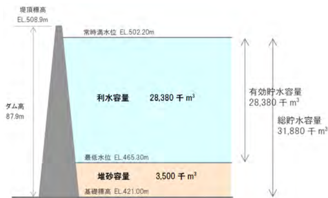
利水専用ダム標準断面図
