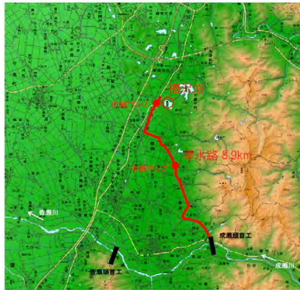
図 導水路ルート図
