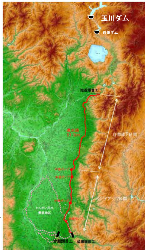
図 導水ルート図
