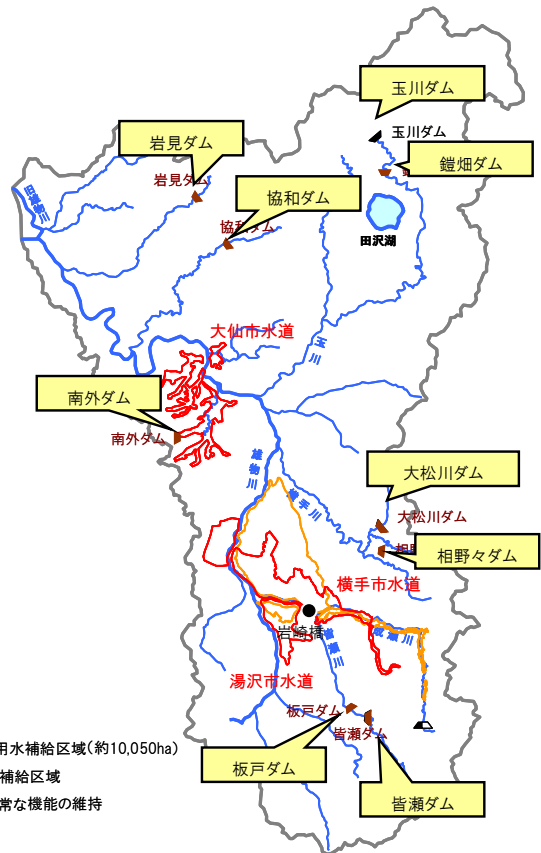
図 4.5-8 既存ダムのかさ上げ・掘削イメージ
