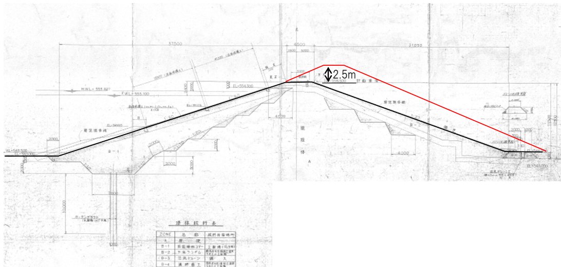
図 ため池かさ上げ断面図
