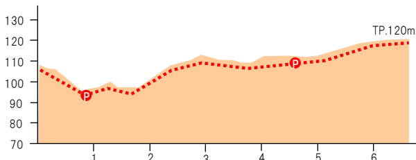
図 導水路縦断面
