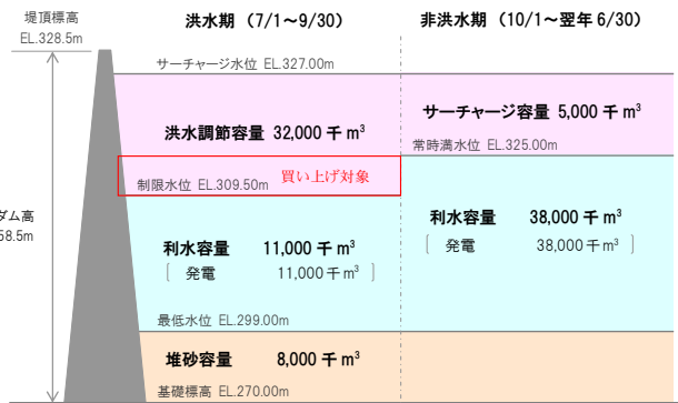
図 鏡畑ダム容量配分図
