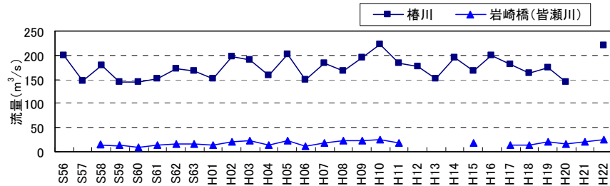
図 2.1-6 主要な流量観測所の平水流量の経年変化
