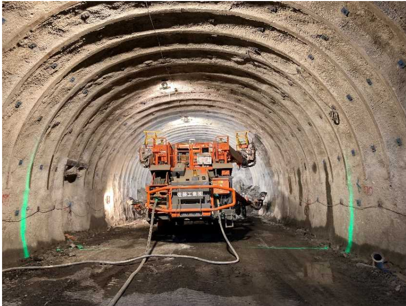
▲ トンネル坑内状況
