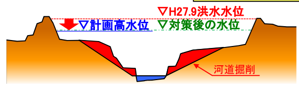
【河道掘削(イメージ)】
