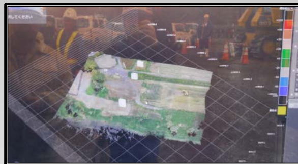
②観測データ点群処理による現況地盤データを確認
