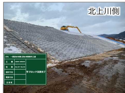
覆土型大型連結ブロック設置状況
