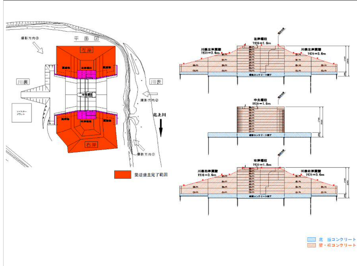
現場配置図
