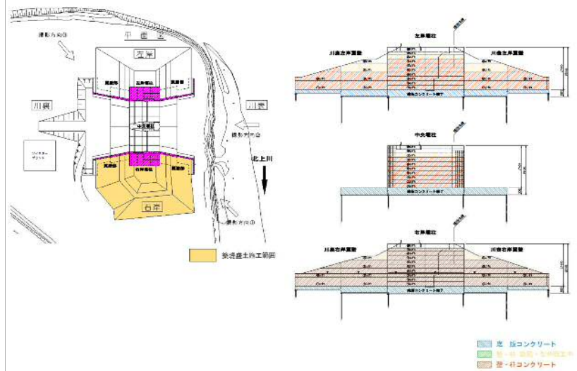
現場配置図
