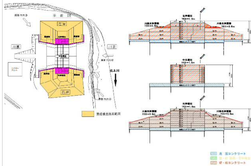
現場配置図
