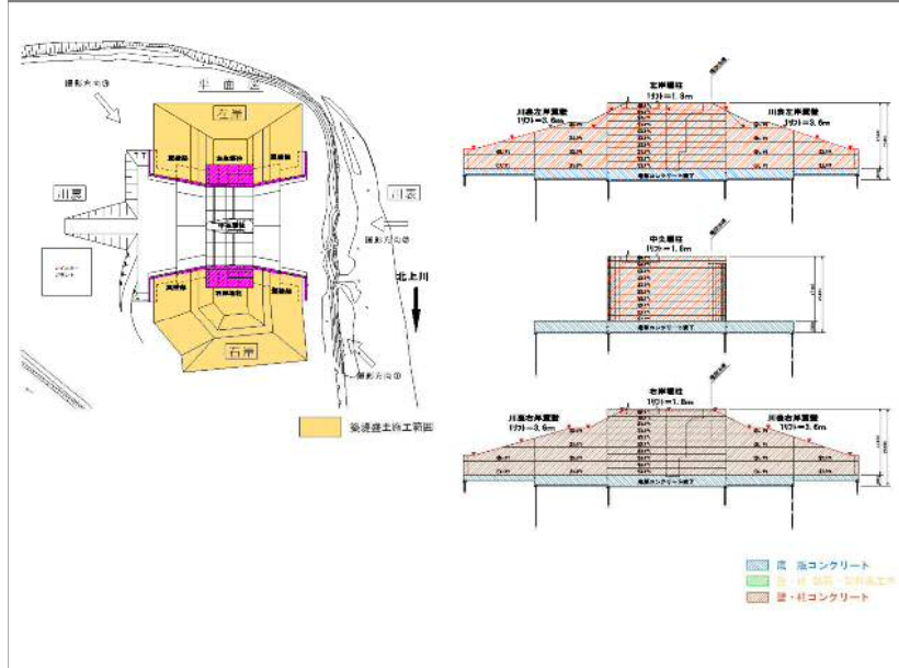
現場配置図
