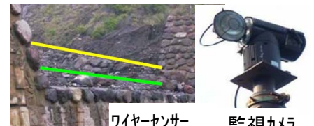
ワイヤセンサー 監視カメラ 監視・観測機器の整備（霧島山（新燃岳））
