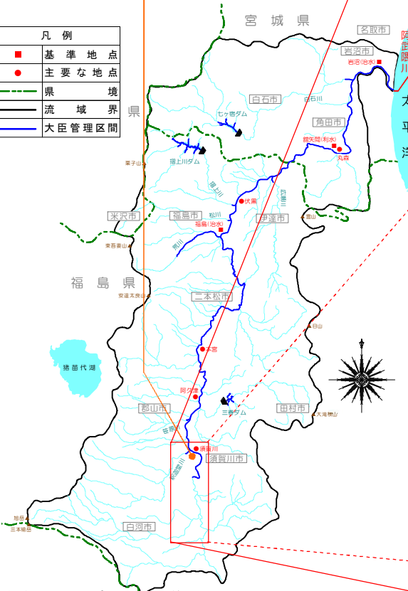
図 5-1-1 遊水地の整備箇所位置図
