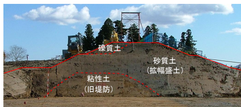
堤防開削断面 (阿武隈川下流 右岸36k付近)
