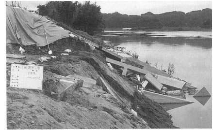
河岸崩壊の状況 昭和 61 年 8 月洪水 宮城県区間 20. 0k 付近
