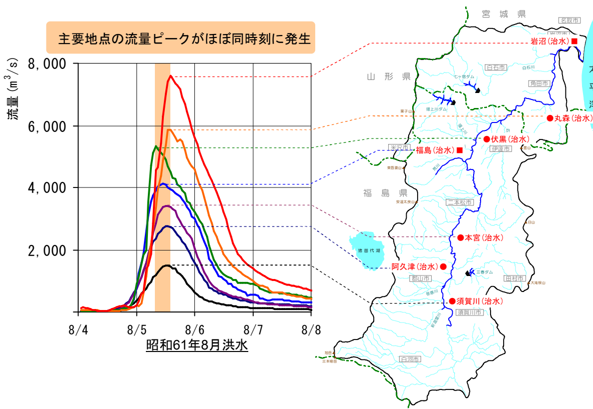
図3-3 阿武隈川水系主要地点の時間一流量曲線【S61.8洪水】
