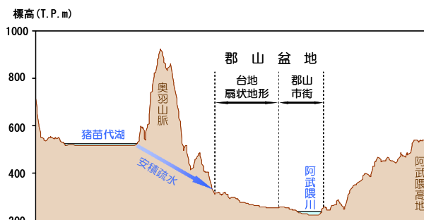
図3-15 猪苗代湖～郡山市の地形模式図
