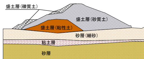
堤防及び基盤の土質イメージ
