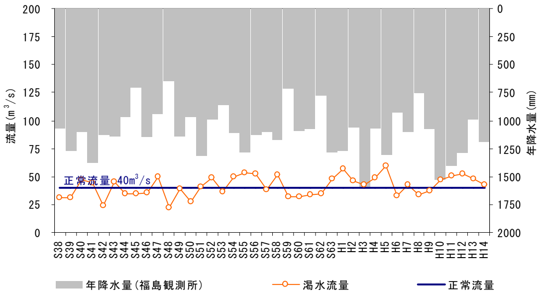
図3-18 館矢間基準点における平水・渇水流量と年降水量(気象庁福島観測所)
