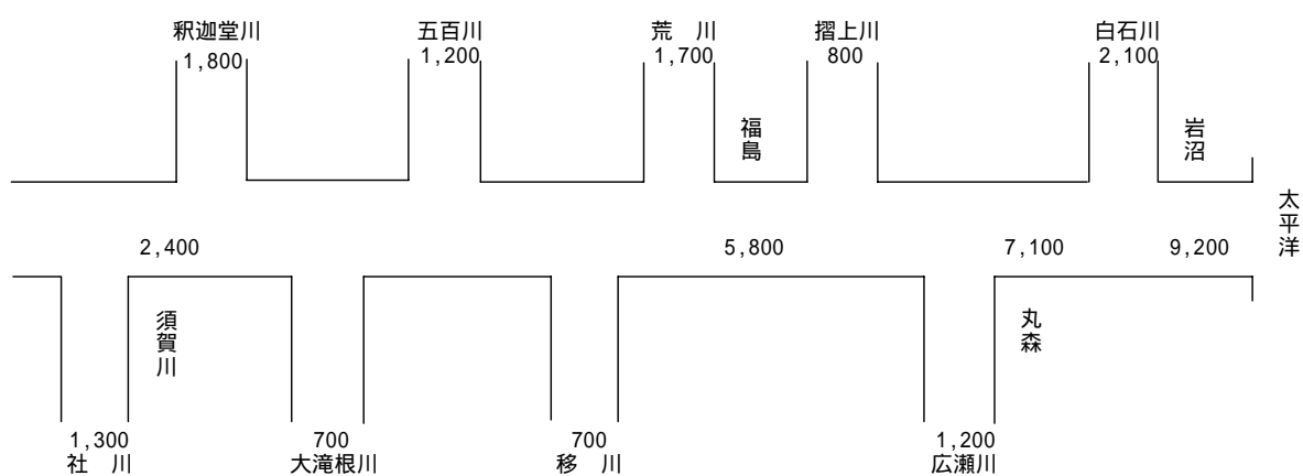
阿武隈川計画高水流量図 (単位：m 3 /s)
